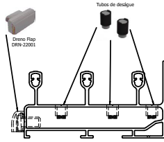
Representação dos Drenos e Tubos de deságue .
