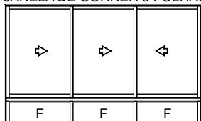
JC302 JANELA DE CORRER 3 FOLHAS COM PEITORIL FIXO
