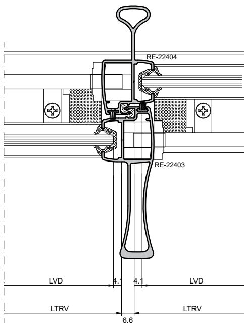
CORTE 04
