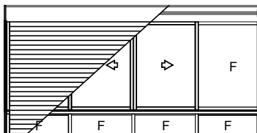
IJC400 JANELA DE CORRER 4 FOLHAS COM PERSIANA INTEGRADA COM PEITORIL FIXO
