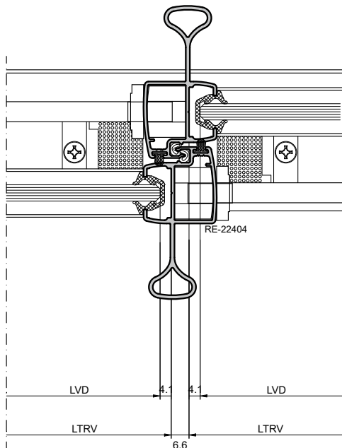
CORTE 04
