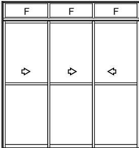
PC301 PORTA DE CORRER 3 FOLHAS COM BANDEIRA FIXA
