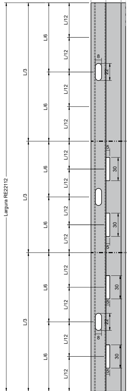
Vista A Esc.: 1:2
