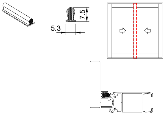
QL-5375 QLON de vedação 5.3x7.5 cor: preto / branco / cinza
