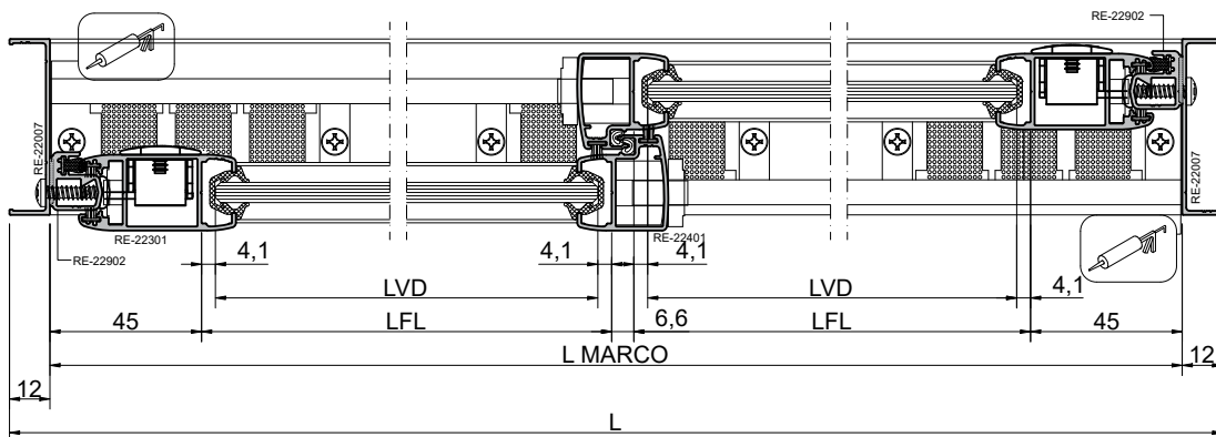
CORTE 03
